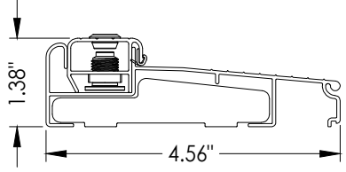
15 INSWING ADJUSTABLE THRESHOLD ZAILAA4565
