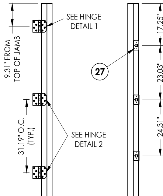
HINGE JAMB
