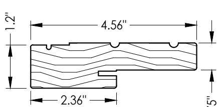
1 WOOD JAMB
